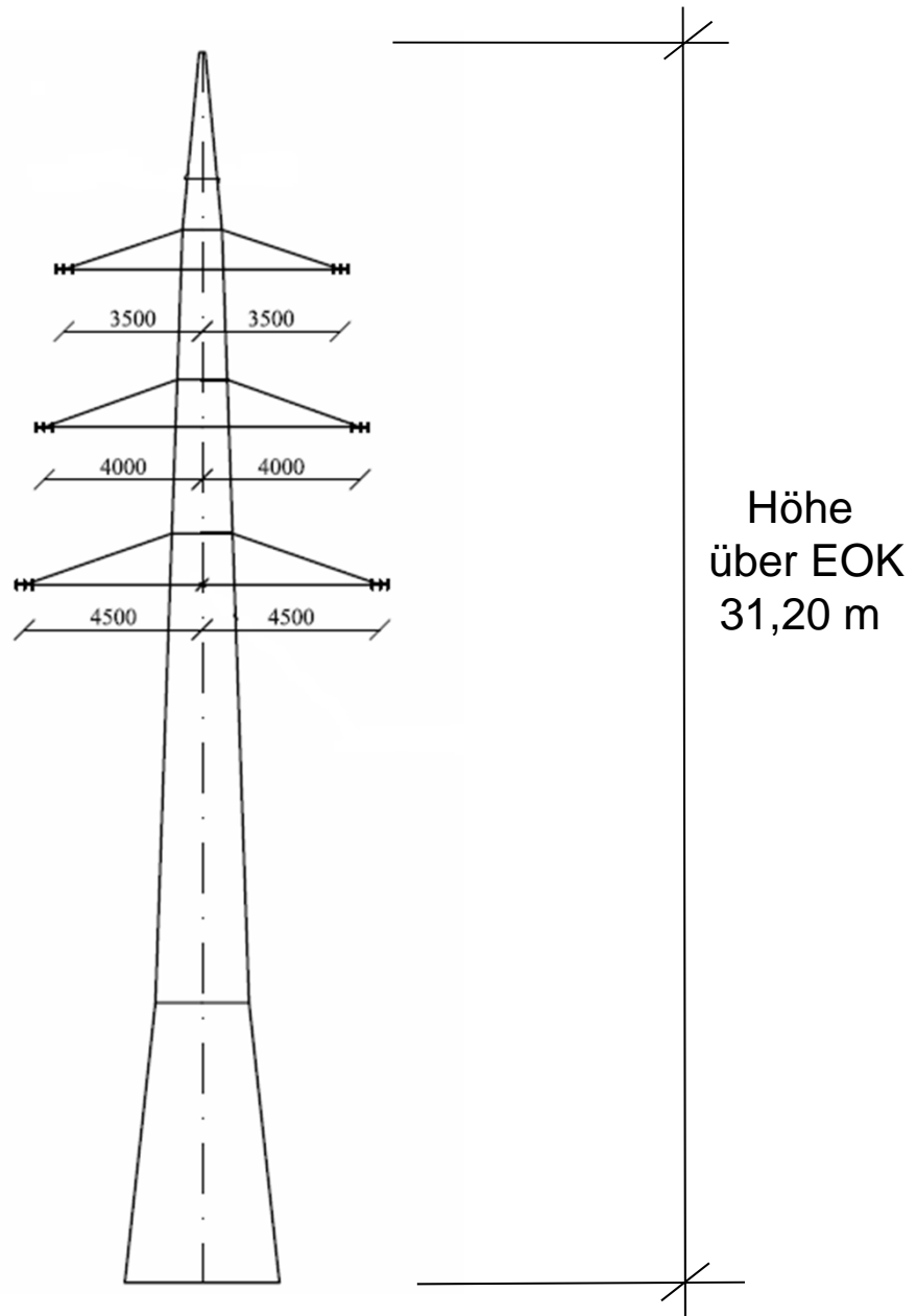
Schemazeichnung (ohne Maßstab) Maßangaben in Meter
