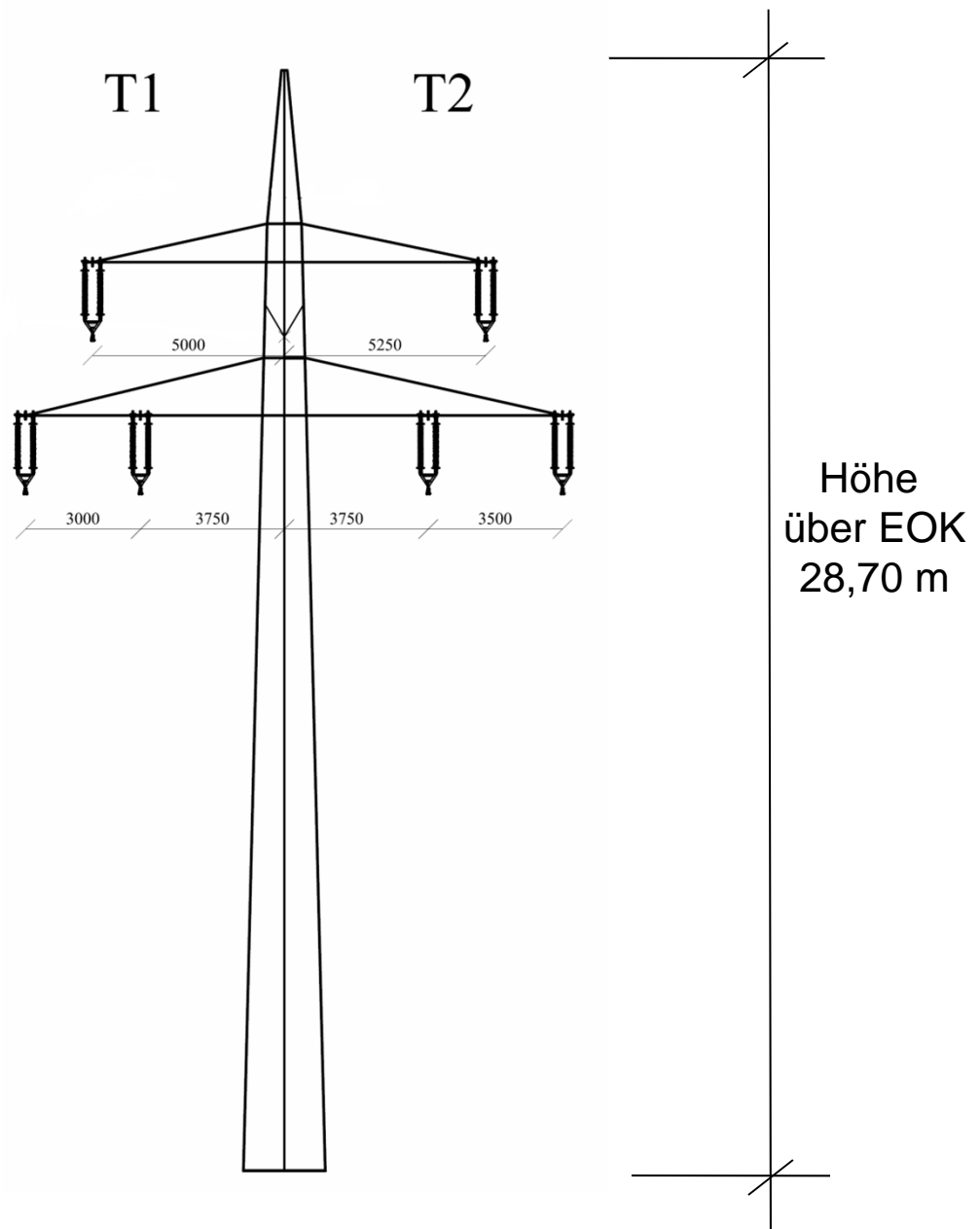
Schemazeichnung (ohne Maßstab) Maßangaben in Meter
